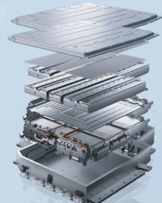
Batería Off-road CATL
