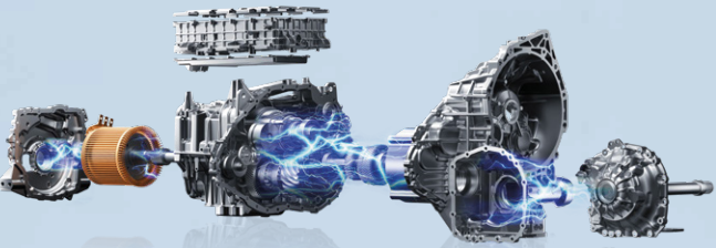
Transmisión longitudinal 2DHT
